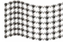
Продольно-поперечная волна
