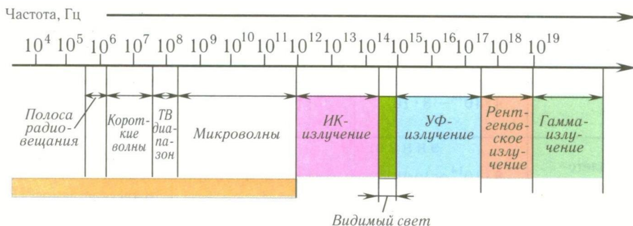
ИК – инфракрасное излучение, УФ – ультрафиолетовое излучение Рис. 1.1 – Спектр электромагнитных волн
