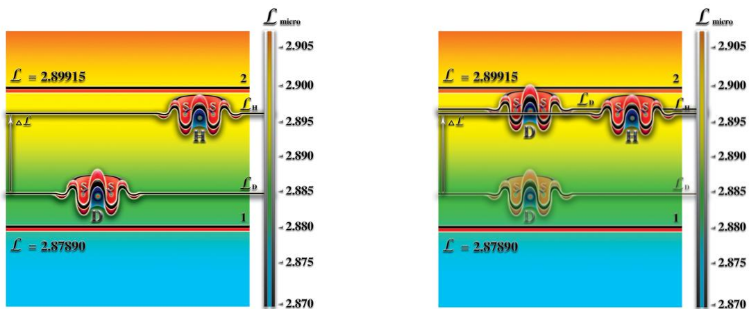
Рис. 1.20 - Радиоактивный изотоп водорода (дейтерий D ) устремляется к оптимальному уровню собственной мерности обычного водорода H
