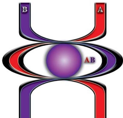
Рис. 1.11 – Слияние двух материй А и В
