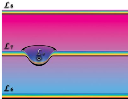
Рис. 1.9 – Нейтронная звезда
