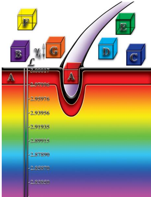
Рис. 1.4 – Мерность различных слоёв пространства и «кубики» материи А, В, С, D, E, F и G
