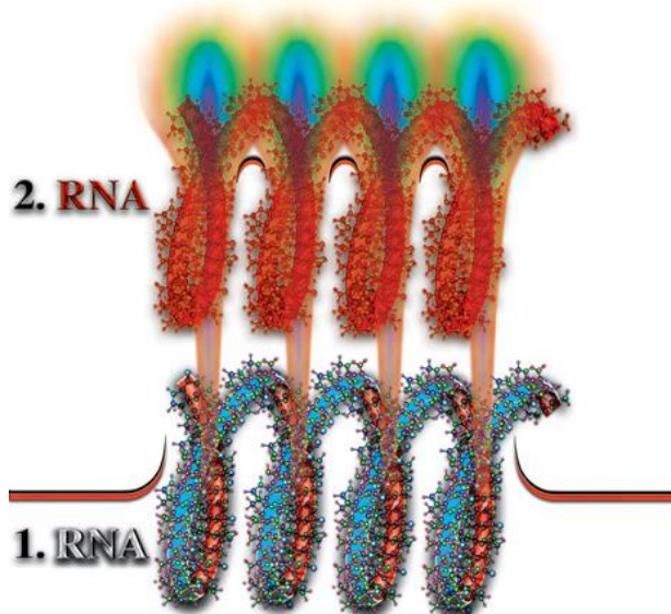
Рис. 2.6 - Формирование на втором материальном уровне копии молекулы РНК - второго материального тела
